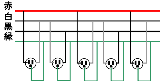
*単相三線式結線(100V)
