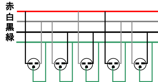
*三相三線式結線(200V)
