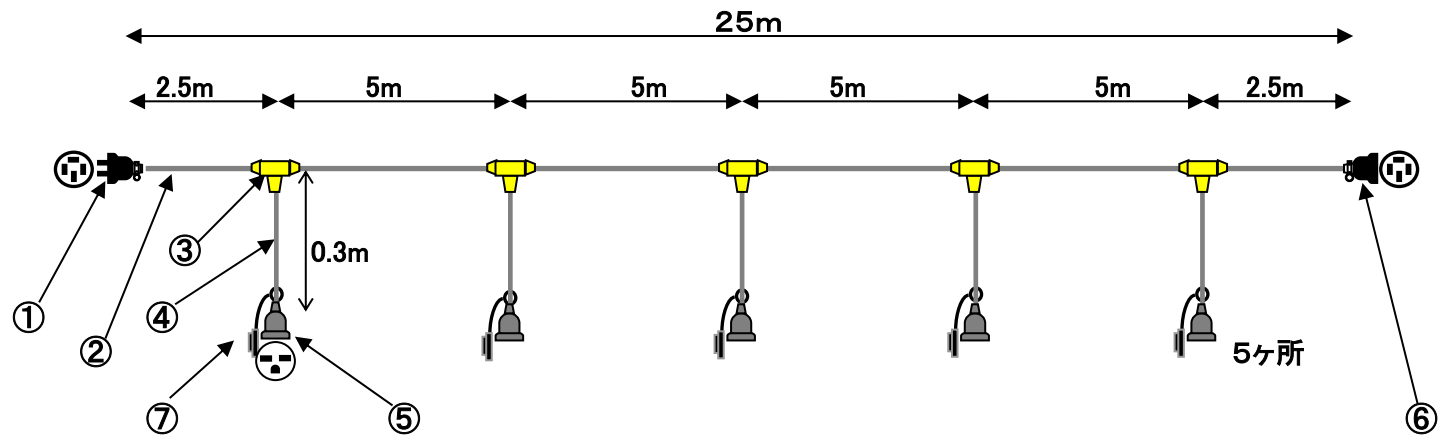
*三相三線式結線(200V)
